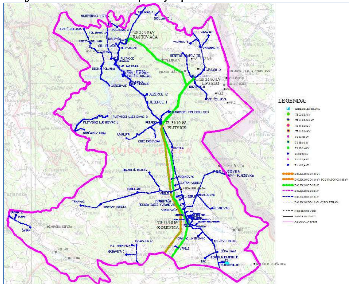
Kartogram 10 - Prikaz SN mreže na području Općine Plitvička Jezera
