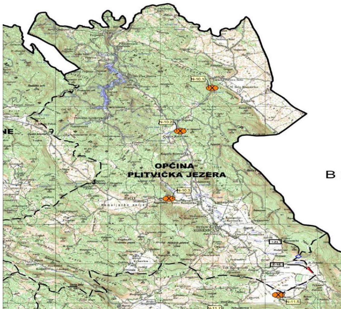
Kartogram 5. – Istraživanje i eksploatacija mineralnih sirovina
